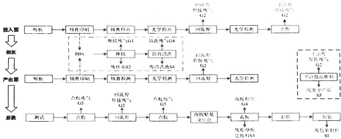
图11 主板生产工艺流程及产污节点图
